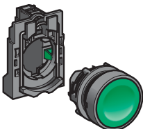
Tryckknappar och omkopplare: kontakthus + manöverhuvud separata enheter
